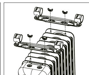
9\11\13 fins heater castor assembly
