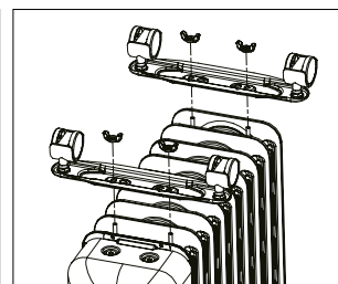
Hjóleining fyrir kynditæki með 9, 11, 13 flönsum.
