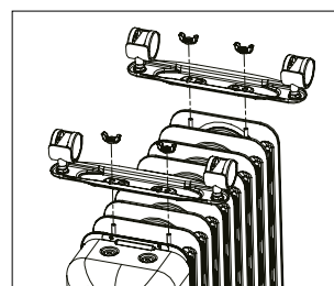
Hjulenhet för värmeelement med 9, 11, 13 flänsar
