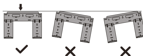
Asennuslevyn oikea kohdistus
