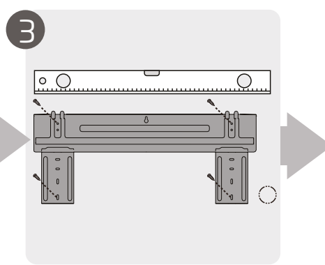
Sett opp monteringsplate
