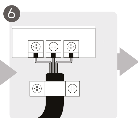
Kople til ledninger
