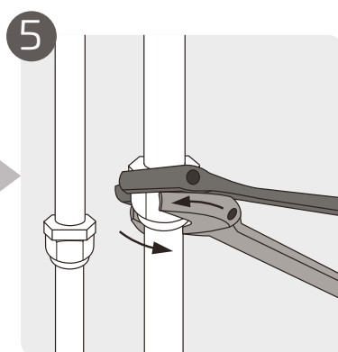
Kople til rør
