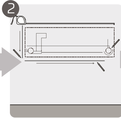
Määritä läpivientiaukon paikka seinässä
