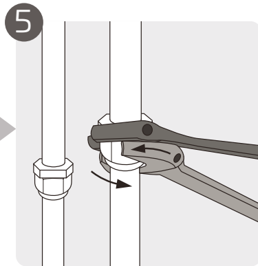
5 Yhdistä putket
