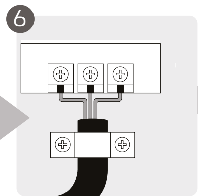
6 Yhdistä sähköjohdot
