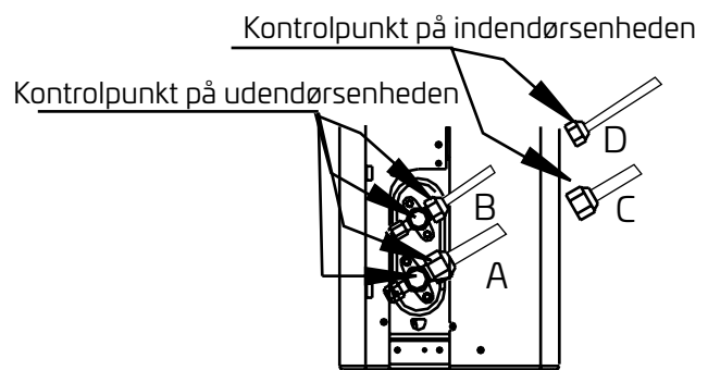
A: Lavtryksstopventil B: Højtryksstopventil C & D: Indendørsenhedens kravemøtrikker
