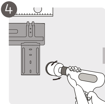
4 Pora läpivientiaukko
