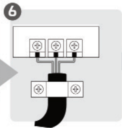
Kople til ledninger (gjelder ikke for enkelte steder i USA)
