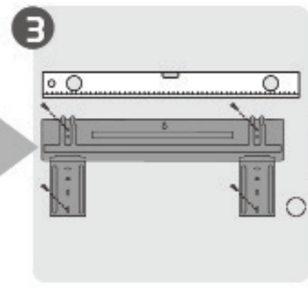
Kiinnitä asennuslevy
