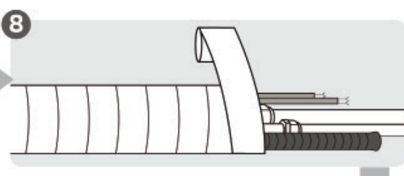
Surr rør og kabel (gjelder ikke for enkelte steder i USA)
