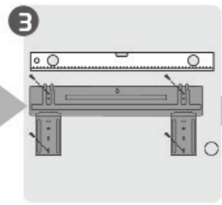
Fäst monteringsplattan
