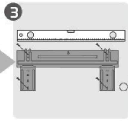
Sett opp monteringsplaten
