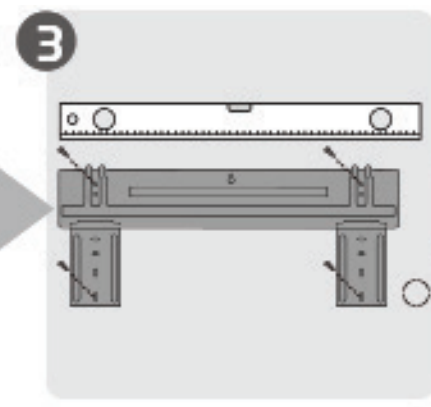
Fastgør monteringspladen
