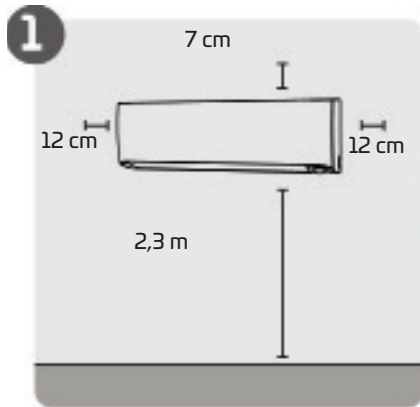
Vælg installationssted
